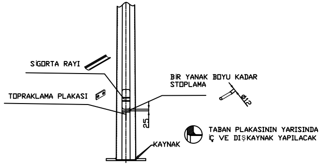
A-A Section
