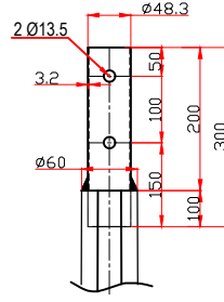
X DETAYI
